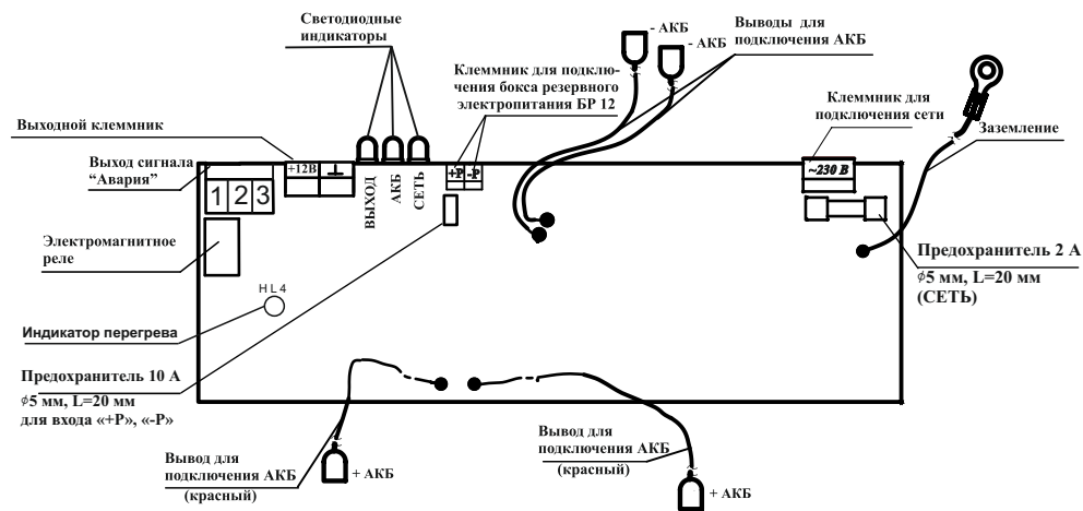
Рисунок 1– Плата источника
