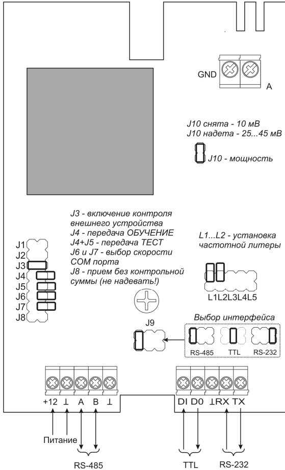
Рис. 2. Монтажная схема передатчика
